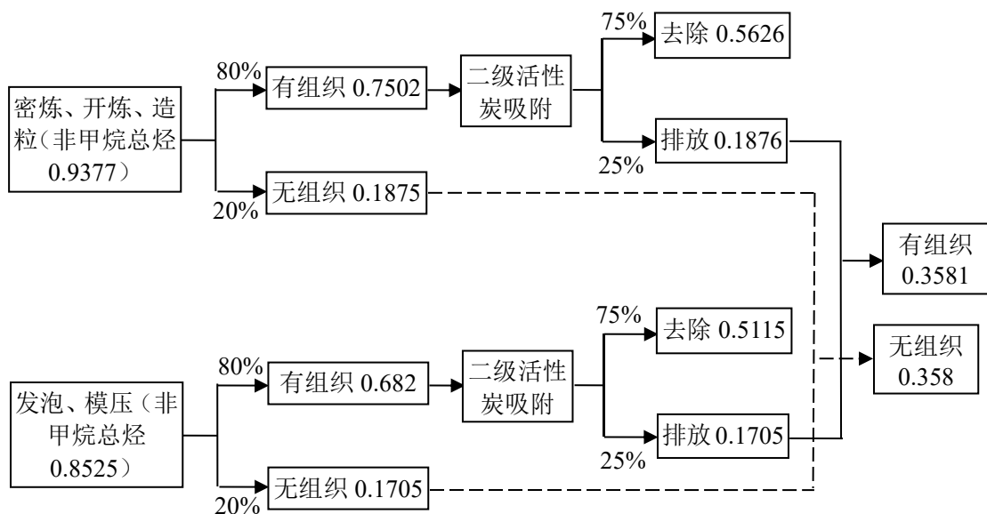
图 2-2 项目物料平衡图（单位：t/a）
