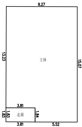
第1层平面图 总面积为:136.67
